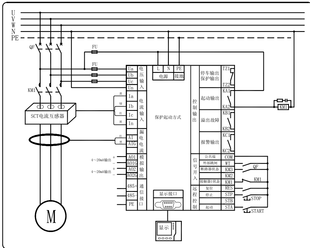
DCM-621M接线原理图（保护方式起动）
