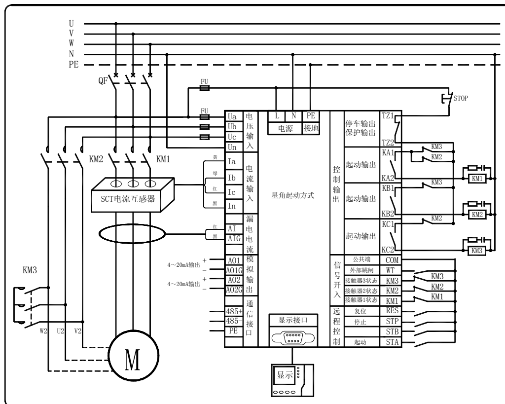
DCM-621M接线原理图（星三角起动）
